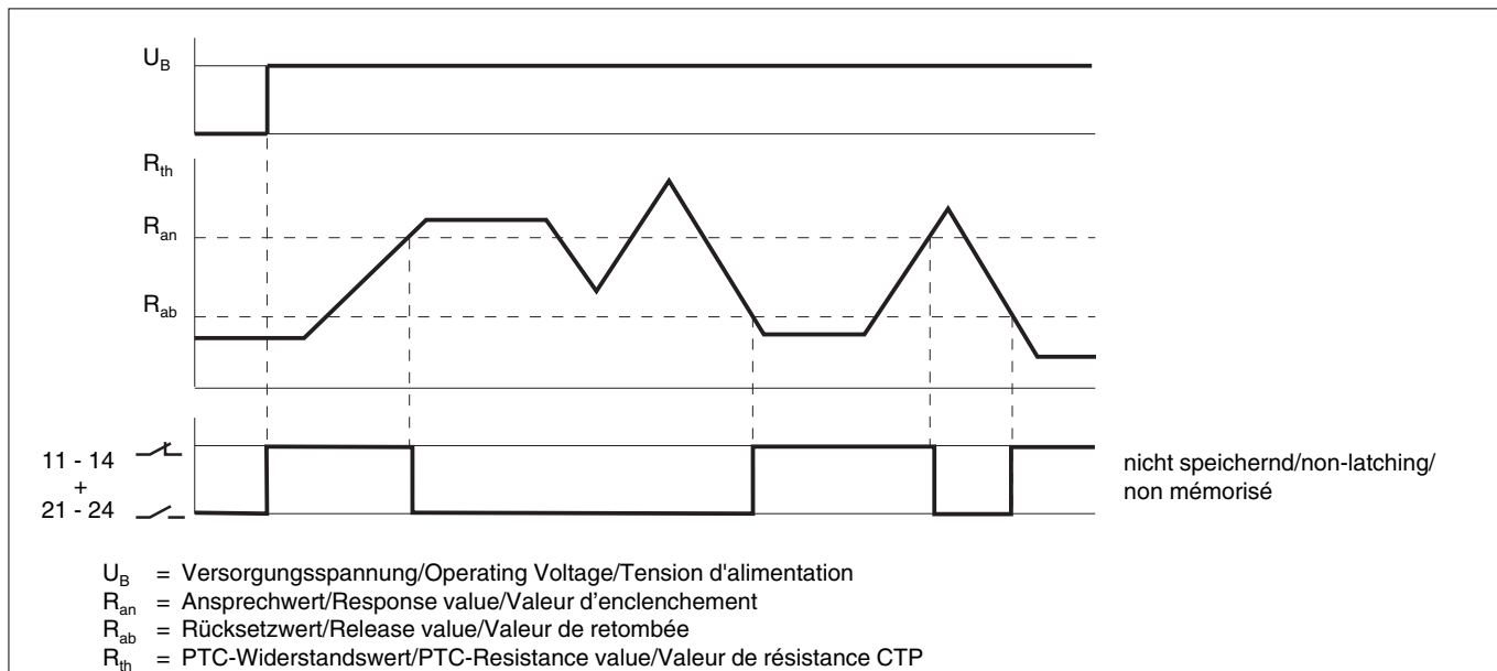
Fig. 2: Funktionsdiagramm
